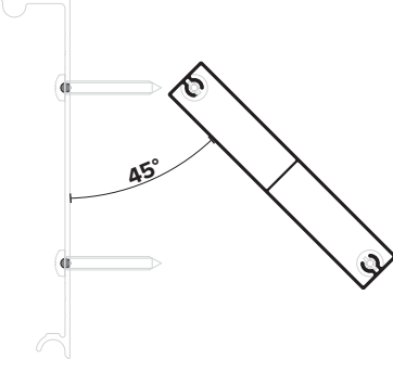
ΚΑΘΕΤΗ ΤΟΜΗ ΜΕ ΚΛΙΣΗ 45°
